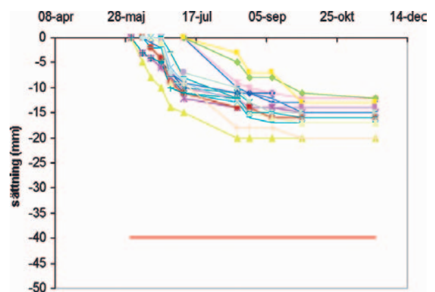
Figur 15: Resultat från sättningsmätningar utförda på pelare i parkeringshuset. Mätningar pågick under hela byggtiden samt tre månader efter färdigställd byggnad.
